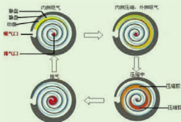
图2 工作原理
